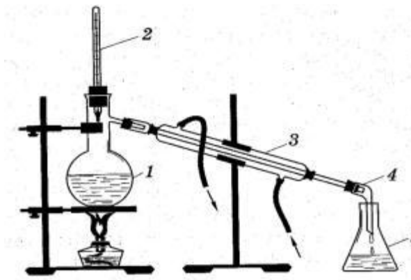
Рис. 2.2. Прибор для прямой перегонки
